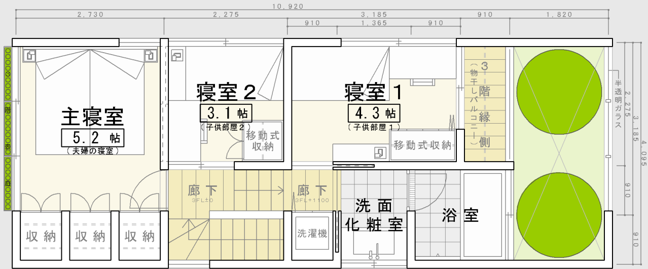
3階平面図
