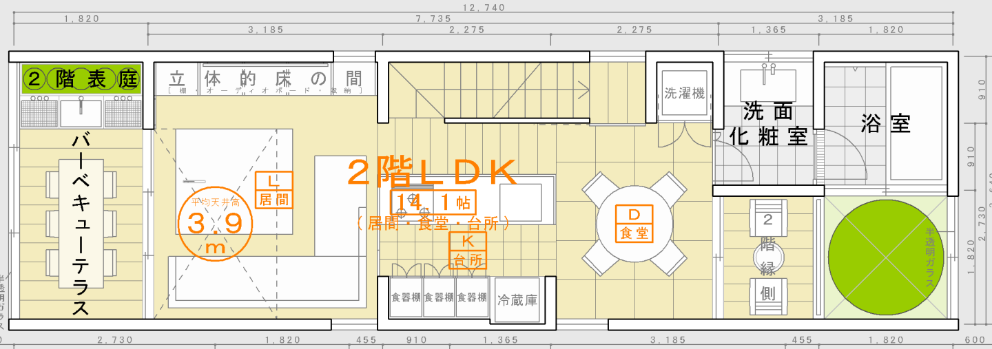
2階にLDKがあります 2階平面図
