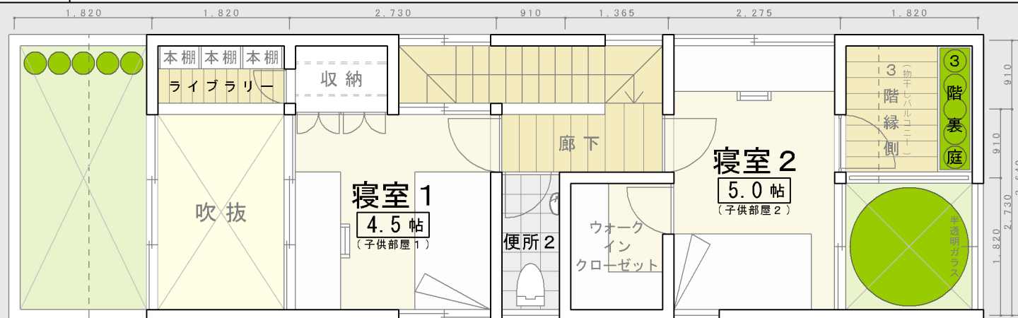
3階平面図
