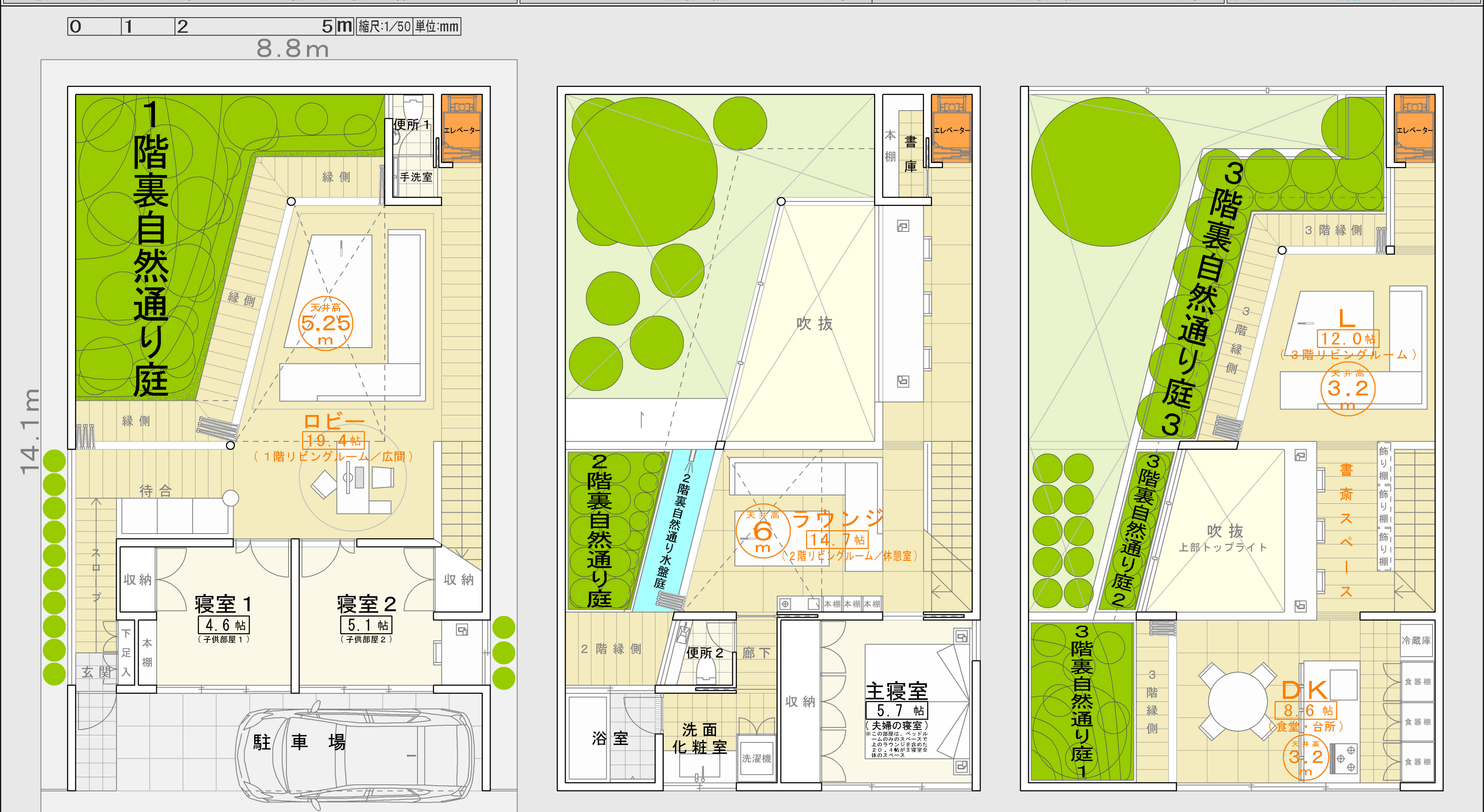
1階1階を真上から見る 2階2階を真上から見る 3階3階を真上から見る
